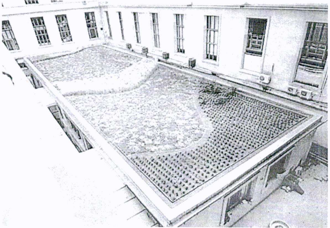
FOTO 1: Vista general de cubierta verde Facultad de Derecho
